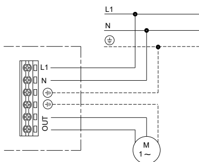
Διάγραμμα καλωδίωσης για μονοφασικές αντλίες
